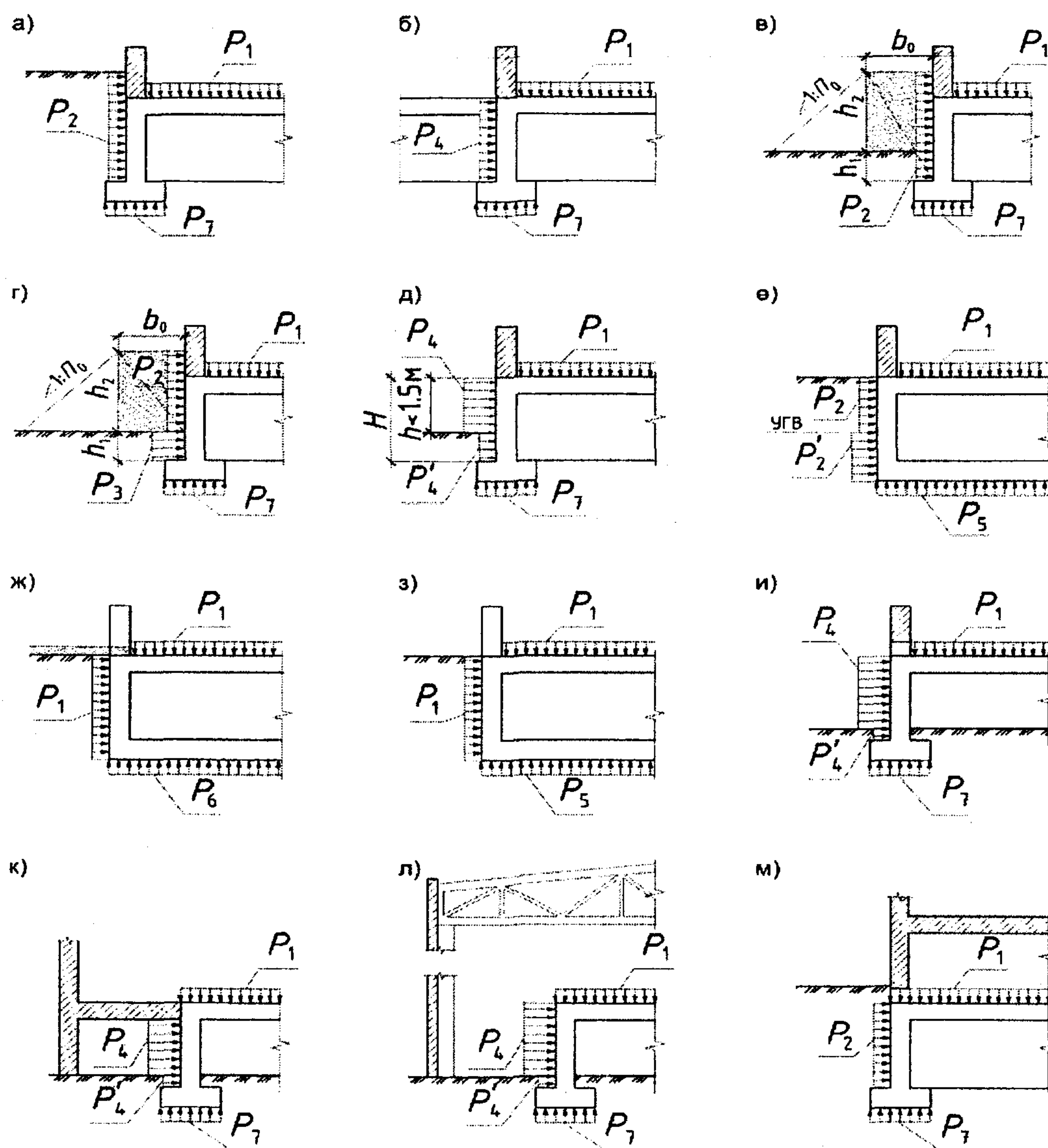
Рисунок 7.1 – Схемы приложения динамических нагрузок на конструкции убежищ
