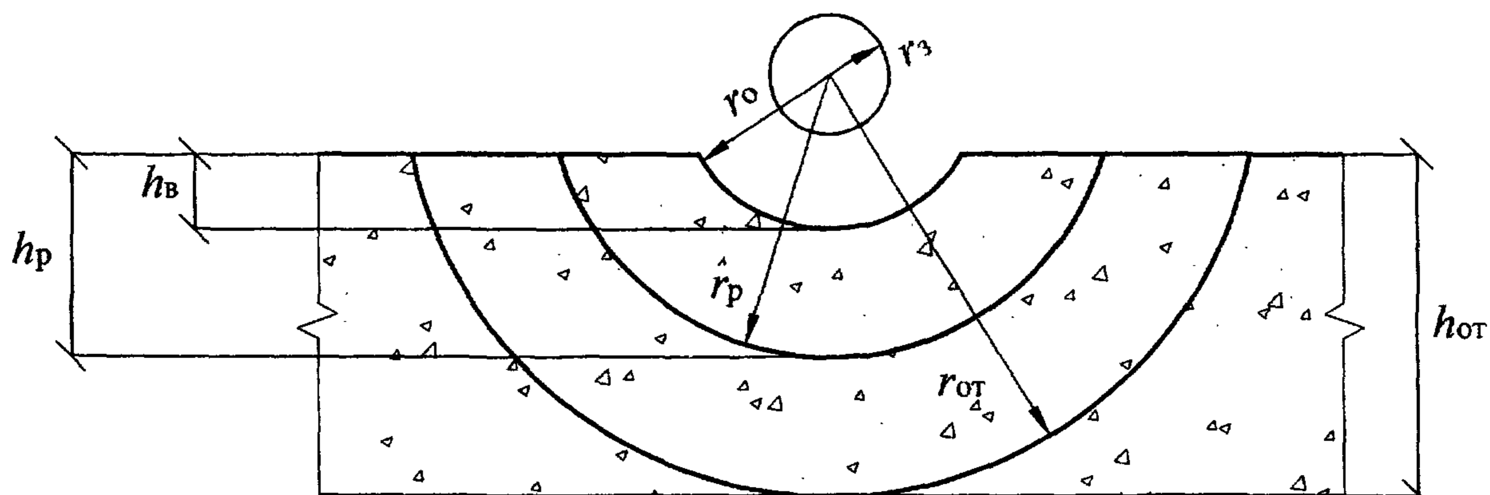
Рисунок Б.2 – Области разрушения преграды при взрыве
