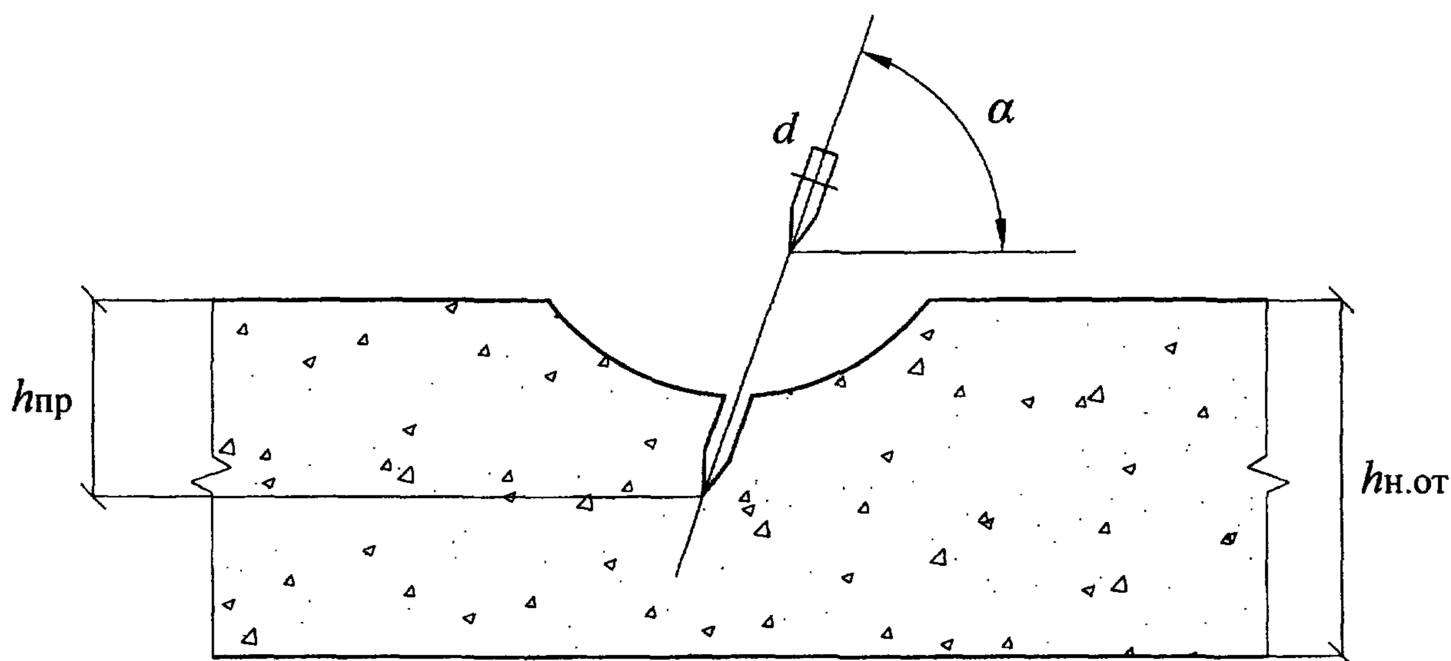
Рисунок Б.1 – Области разрушения преграды при ударе
